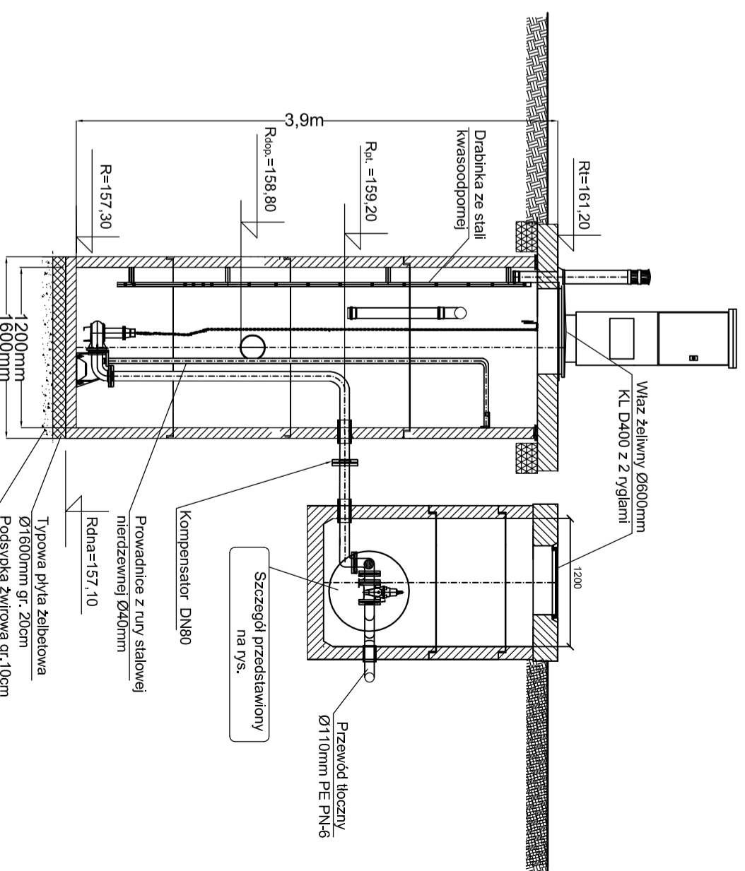
PRZEKRÓJ B-B
