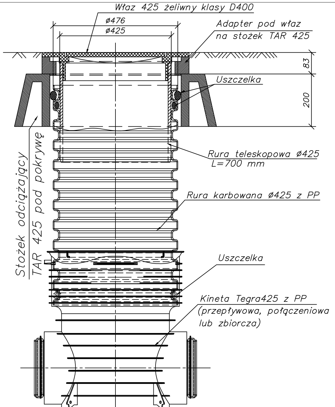
Studzienka inspekcyjna 425 z rurą teleskopową i włazem żeliwnym KL D400 na stożku odciążającym TAR 425
