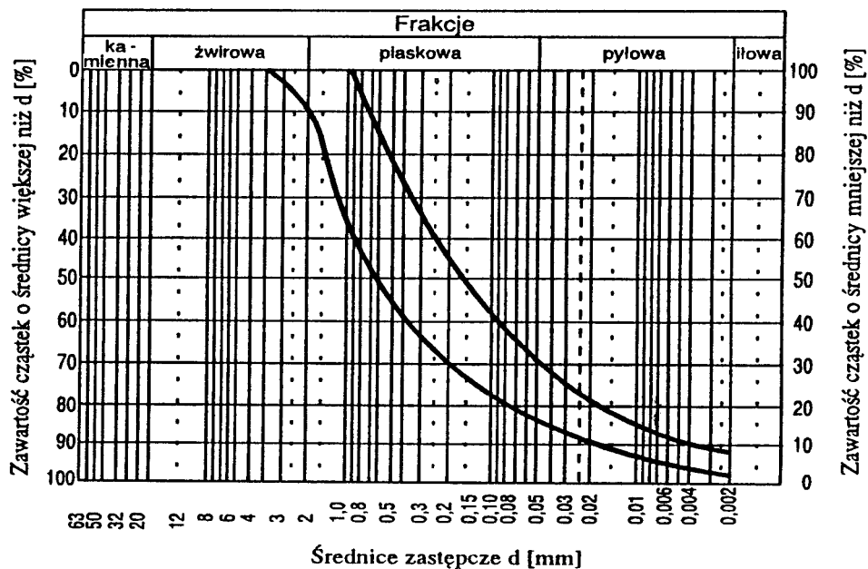
Rys. 1. Obszar uziarnienia optymalnej mieszanki gliniasto-piaskowej
