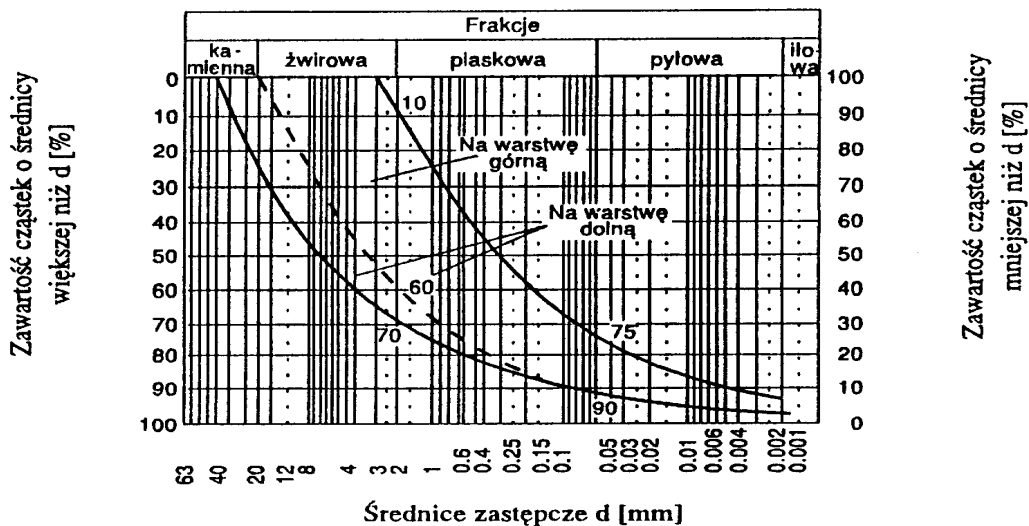
Rys. 2. Obszar uziarnienia optymalnej mieszanki gliniasto-żwirowej
