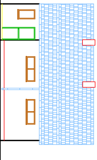
ELEWACJA PÓLNOGNO - WSCHODNIA
