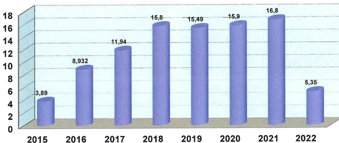
Wykres nr. 10 Długość przebudowanych i wybudowanych dróg w Gminie Dobre w latach 2015-2021 wyrażona w km (drogi asfaltowe oraz stabilizacje cementowe)
