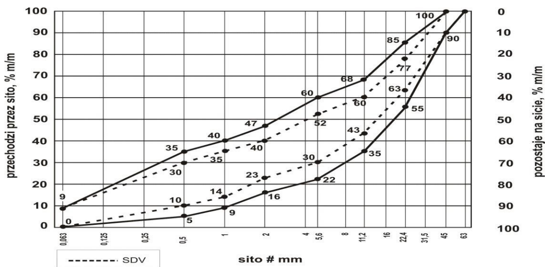
Rys. 6. Uziarnienie mieszanki niezwiązanej 0/63 dla podbudowy zasadniczej
