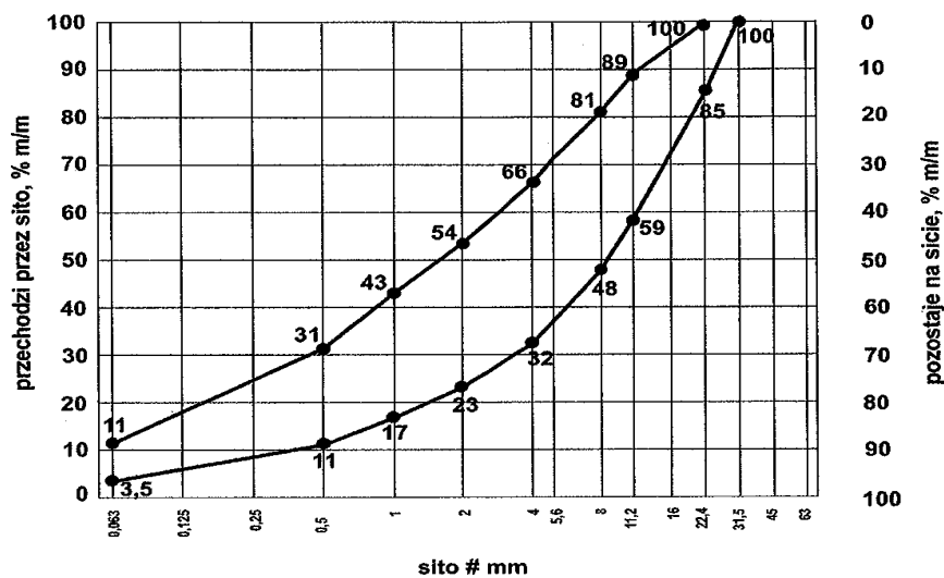
Rys. 2. Krzywe graniczne uziarnienia mieszanki mineralnej 0/22,4 mm
