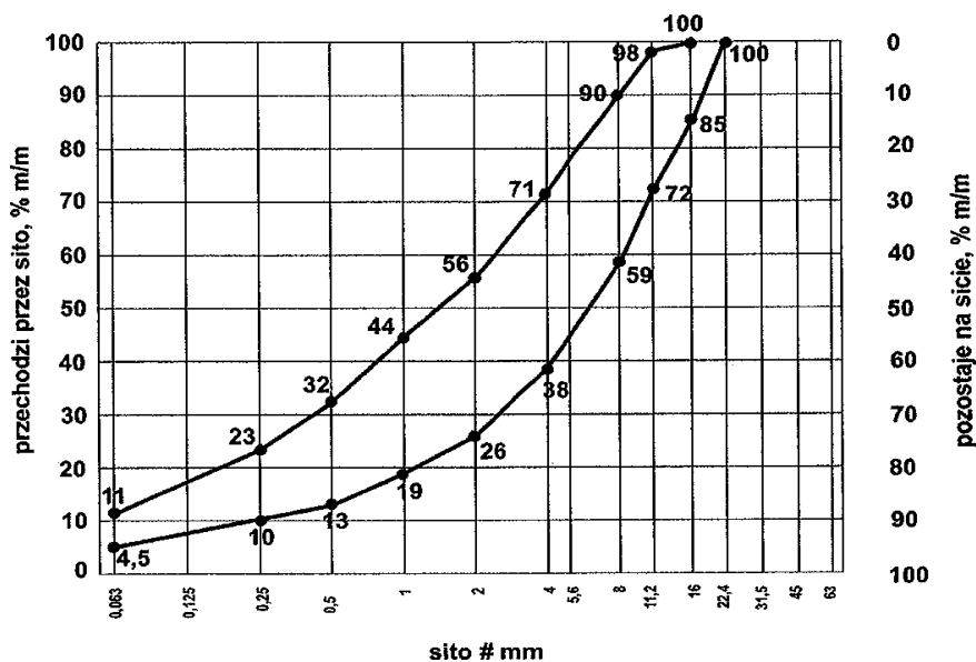
Rys. 3. Krzywe graniczne uziarnienia mieszanki mineralnej 0/16 mm
